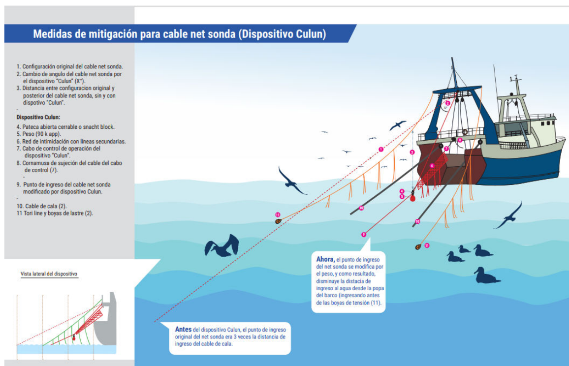
Figura 1. Despliegue de sistema "Culun" con patea y pesos flotantes en reemplazo de patea fija
